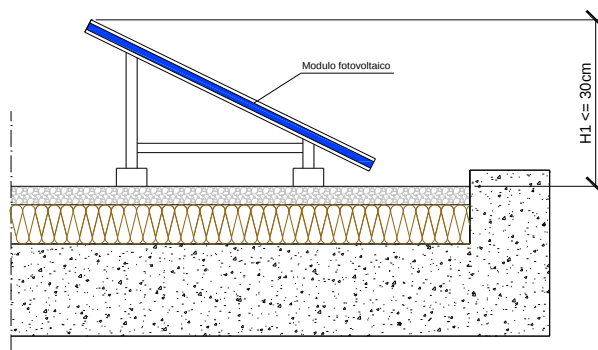
Figura 1 - Caso 1, H \leq 30\text{cm} - Schema esemplificativo di un'installazione idonea alla classificazione dell'impianto fotovoltaico nella categoria "su edifici"
