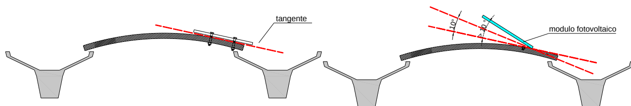
Figura 12 – Schema esemplificativo di una corretta installazione: complanarità al piano tangente o ai piani tangenti del tetto, con una tolleranza di più o meno 10 gradi.
